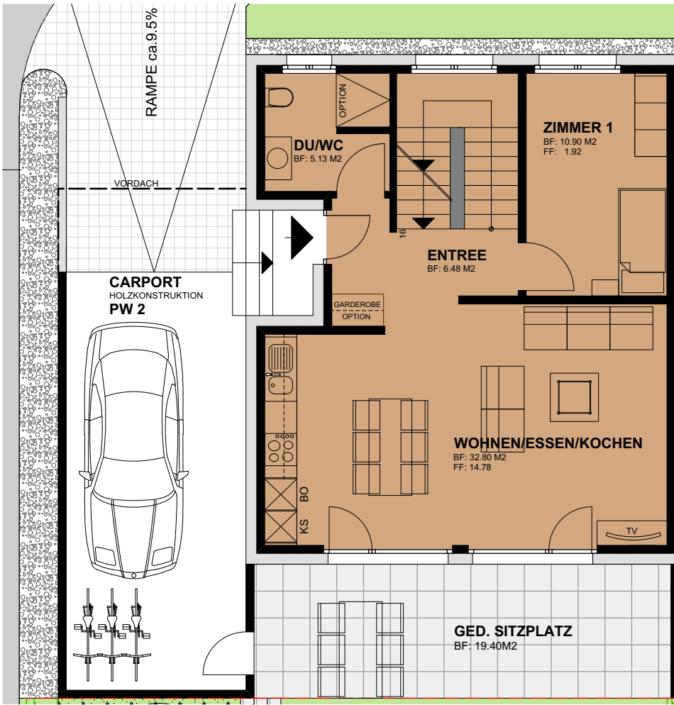
ERDGESCHOSS
