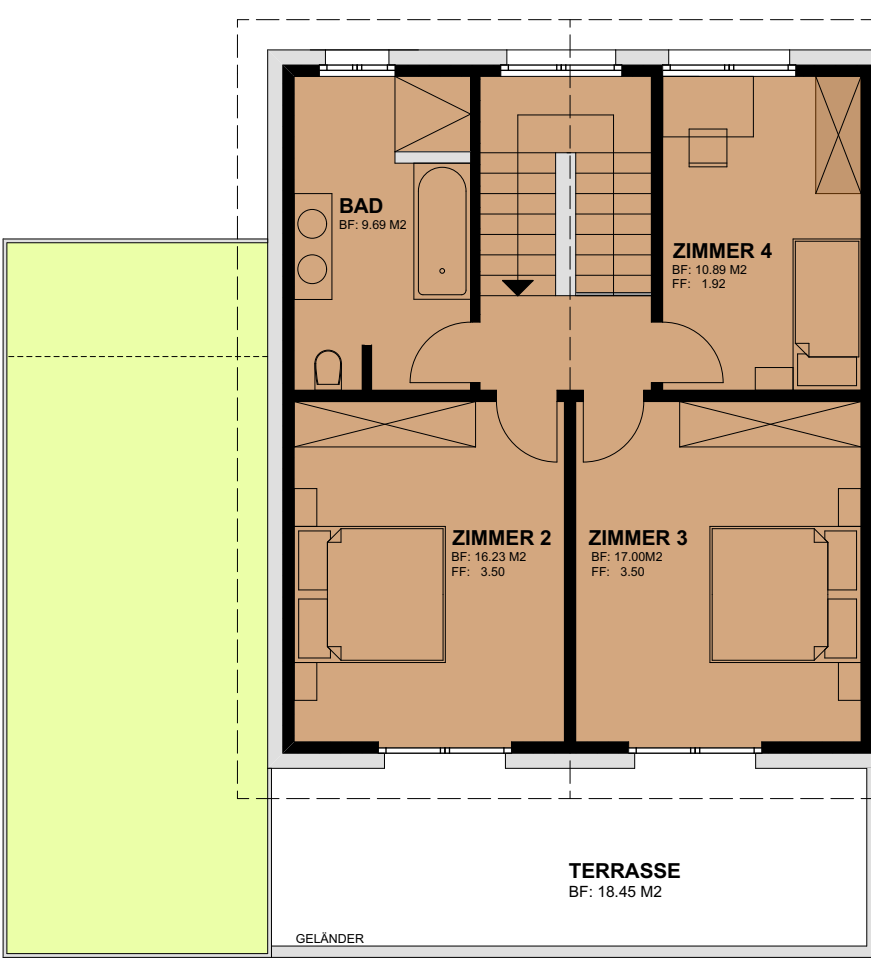
OBERGESCHOSS
