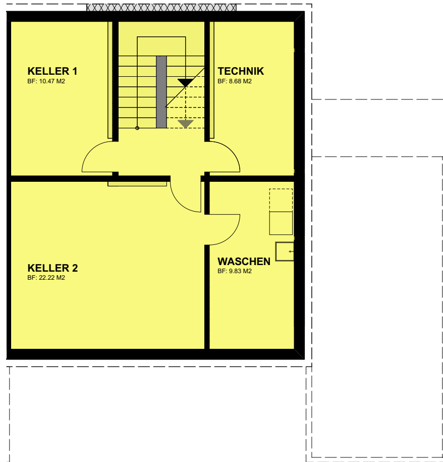
UNTERGESCHOSS
