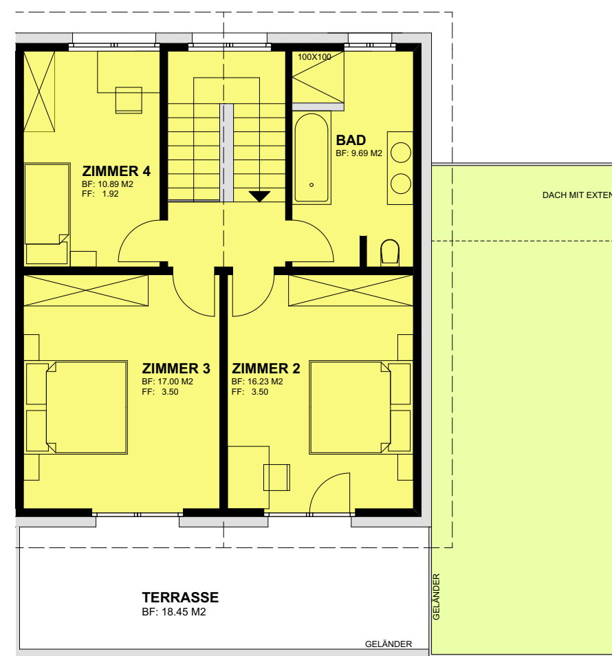
OBERGESCHOSS
