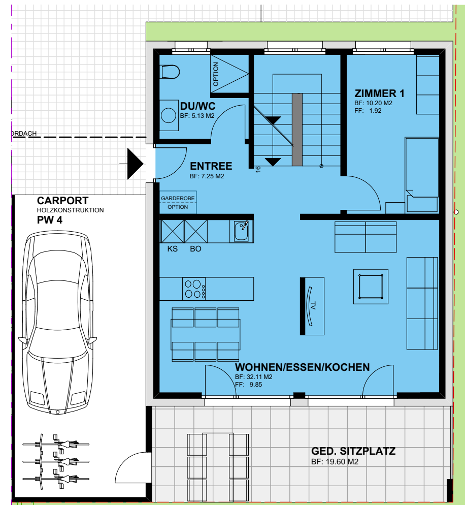
ERDGESCHOSS
