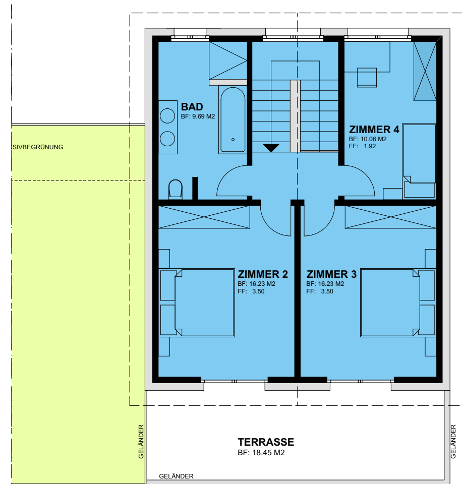
OBERGESCHOSS
