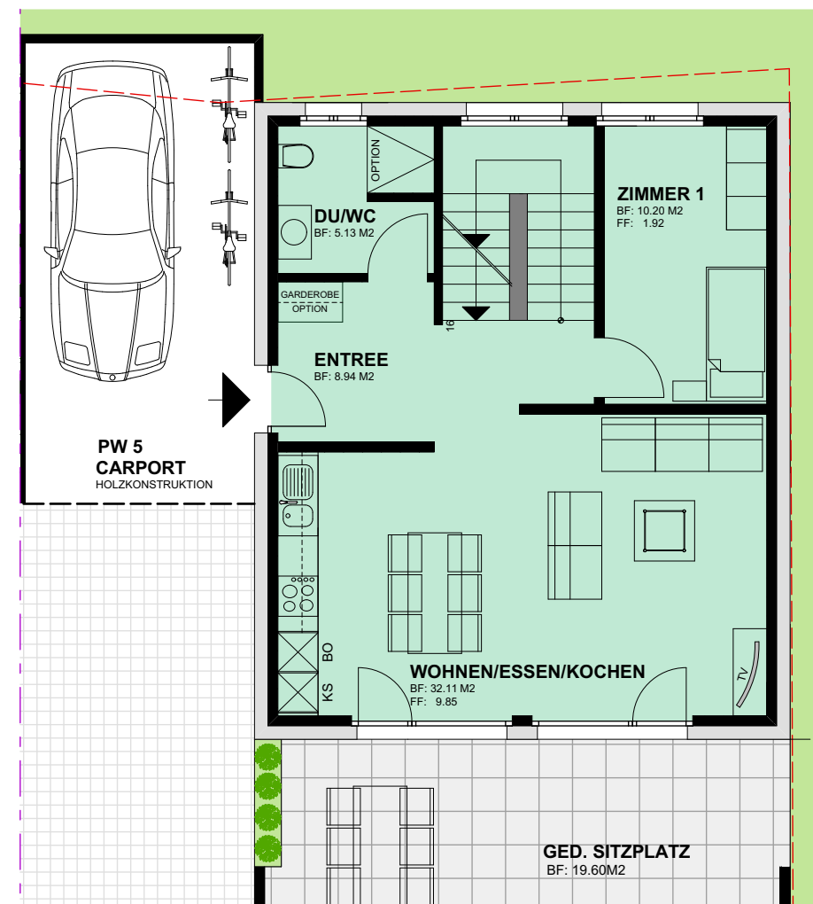
ERDGESCHOSS
