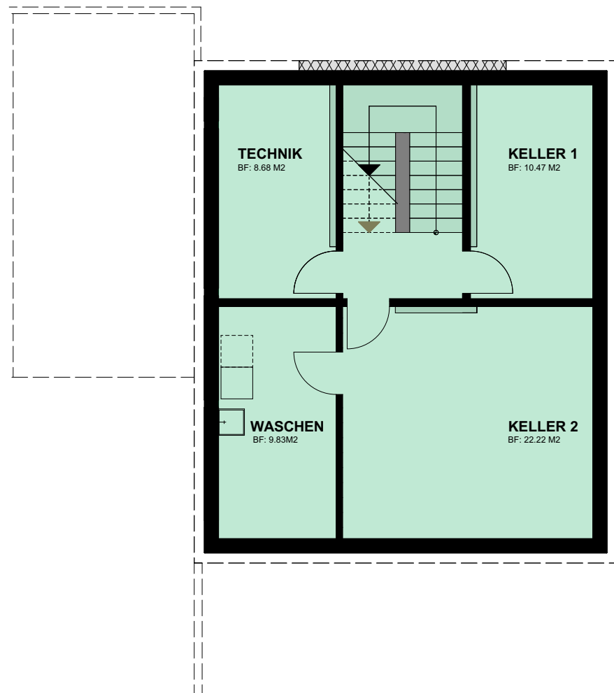
UNTERGESCHOSS
