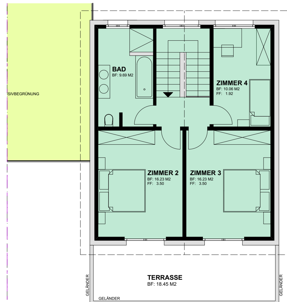
OBERGESCHOSS
