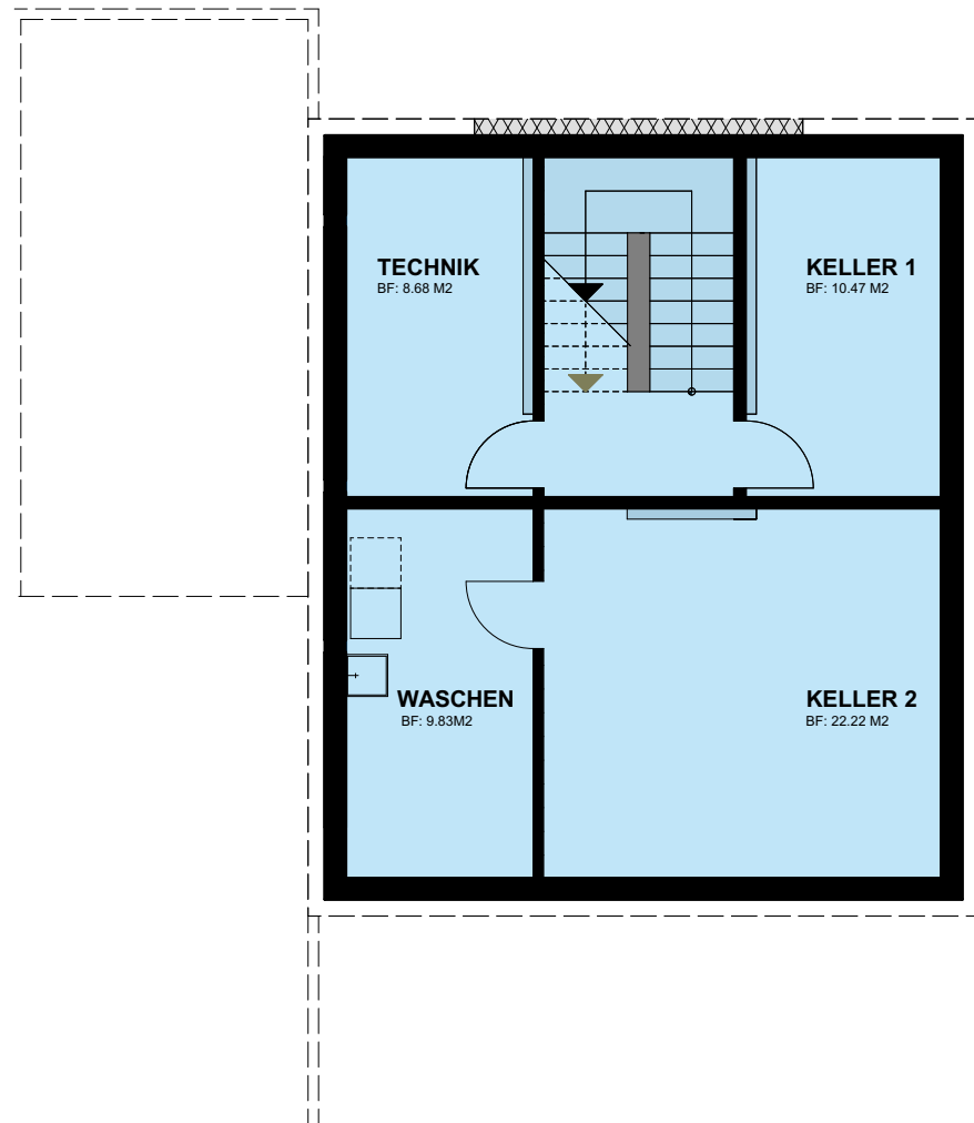
UNTERGESCHOSS
