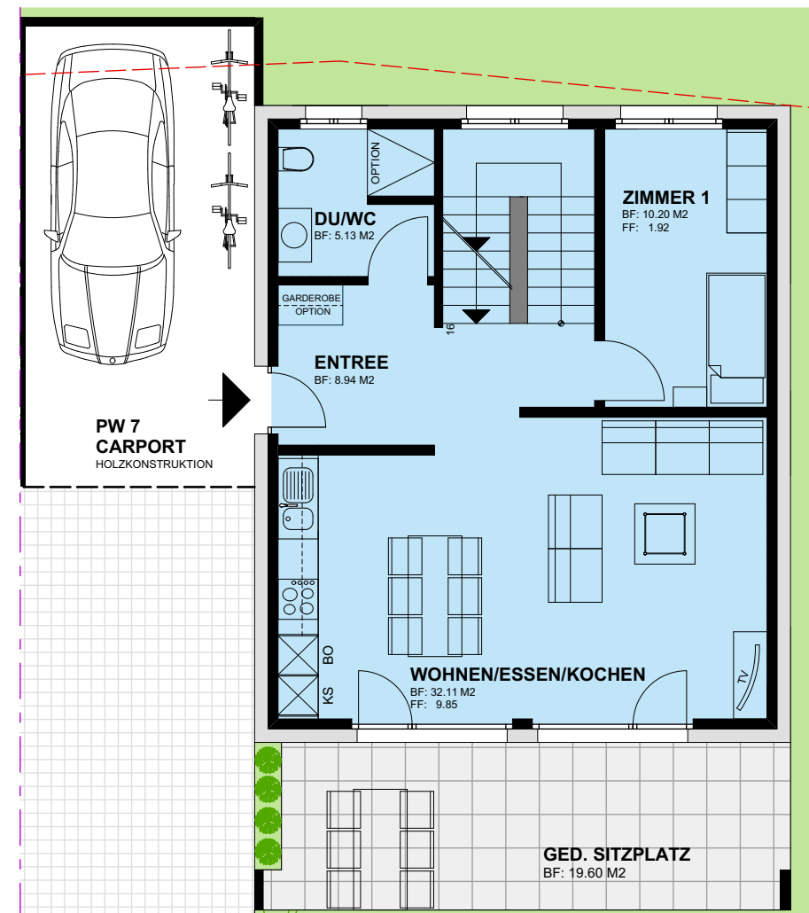
ERDGESCHOSS
