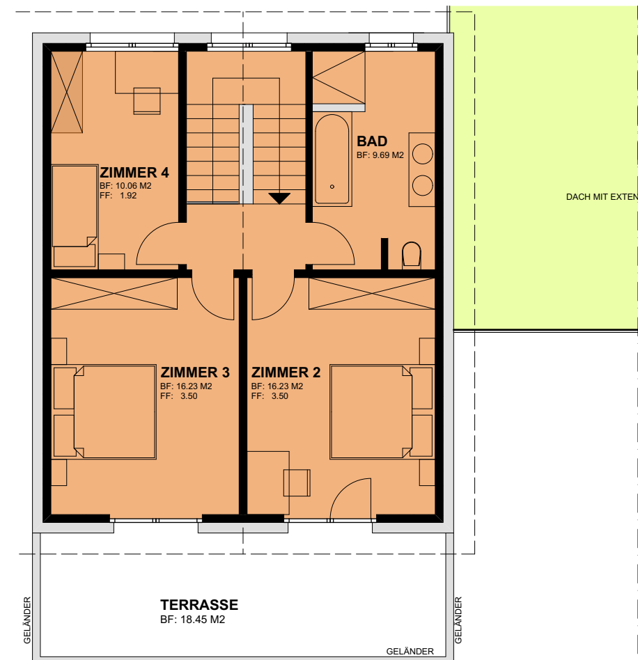
OBERGESCHOSS
