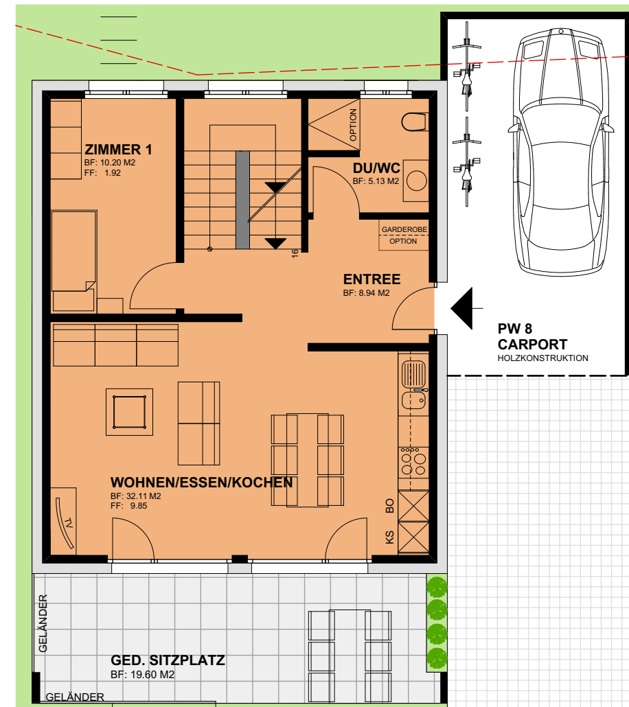
ERDGESCHOSS
